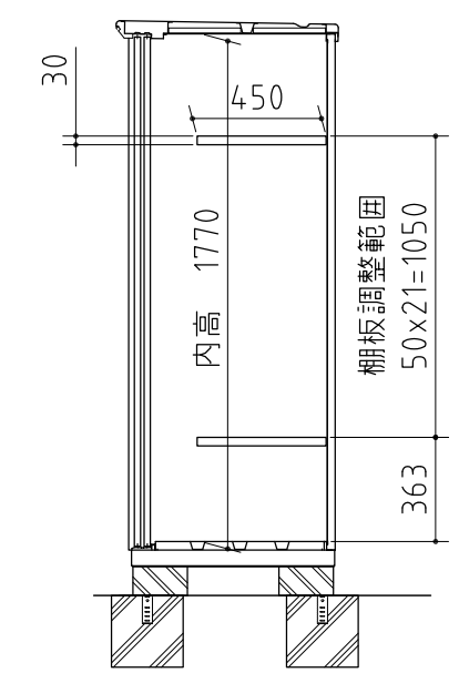
断面図
