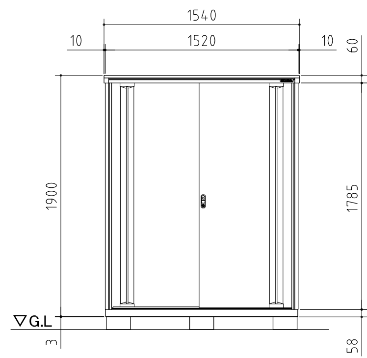
正面図
